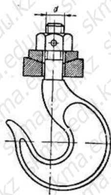
Рисунок 10.7 – Грузовой крюк
